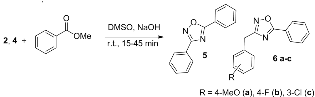
Рис. 2. Схема синтеза 3,5-дизамещенных оксадиазолов из амидоксимов
