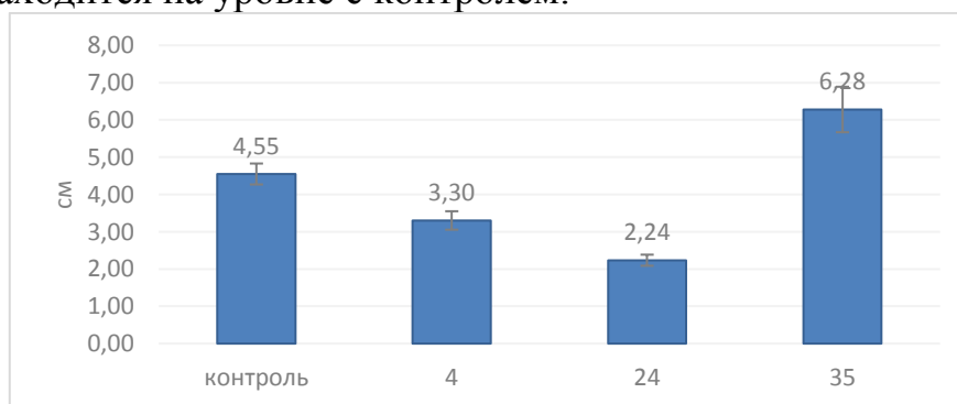
Рис. 2. Влияние на рост листьев Zea mays L. штамма Pseudomonas 16 Н, культивируемого в различных температурных режимах
