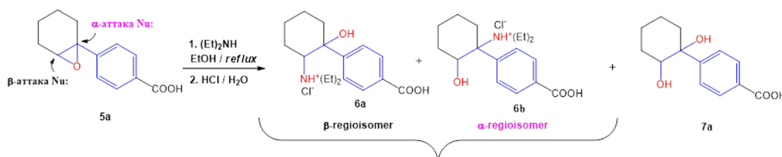
Рис. 2. Взаимодействие 4-пергидро-1-бензоксирен-1-илбензойной кислоты ( 5a ) с N,N -диэтиламином
