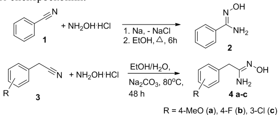
Рис. 1. Схемы синтеза бензамидоксима и амидоксимов бензильного типа из нитрилов
