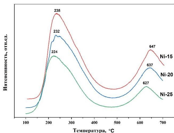
Рис.1. TPD- \text{CO}_2 профили образцов прокаленных СДГ состава \text{Mg}/\text{AlNiX} с различной степенью замещения алюминия на трехвалентный никель X: 1- \text{Mg}/\text{AlNi15} , 2- \text{Mg}/\text{AlNi20} , 3- \text{Mg}/\text{AlNi25}
