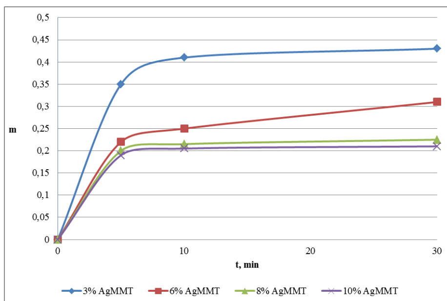
Рис. 1. Кинетика высвобождения ионов коллоидного серебра
