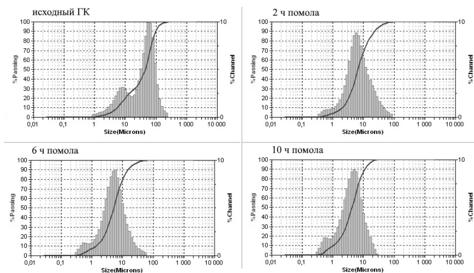
Рис. 1. Интегральная кривая и гистограмма распределения частиц по размерам исходного ГК и продуктов его измельчения в шаровой мельнице
