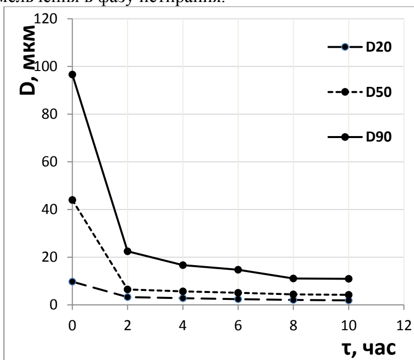
Рис 1. Кинетические кривые процесса измельчения ГК-1
