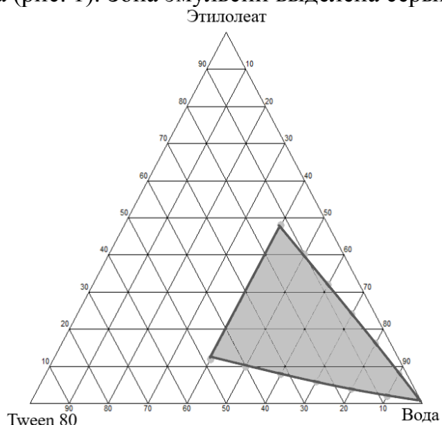
Рис.1. (Псевдо)троичная фазовая диаграмма
