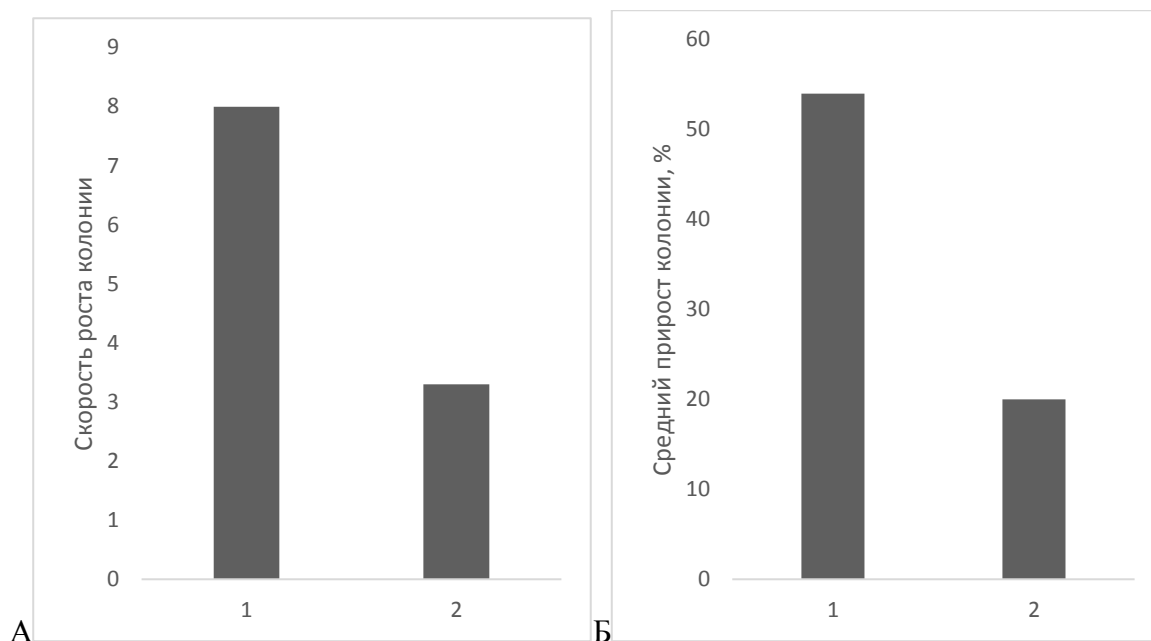
Рис. 1. Скорость роста (А) и средний прирост (Б) колонии A. inguis ВКМ F-1754 как показатель антагонистического потенциала ВКРЛ5
