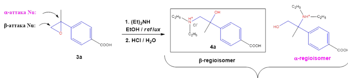
Рис. 1. Взаимодействие 4-(2-метил-2-оксиранил)бензойной кислоты ( 3a ) с N,N -диэтиламином
